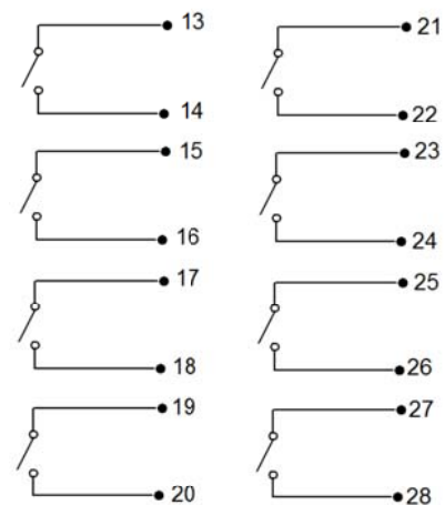
Rys. 12. Wyjścia przekaźnikowe.
