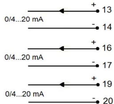
Rys.15. Wyjścia analogowe.
