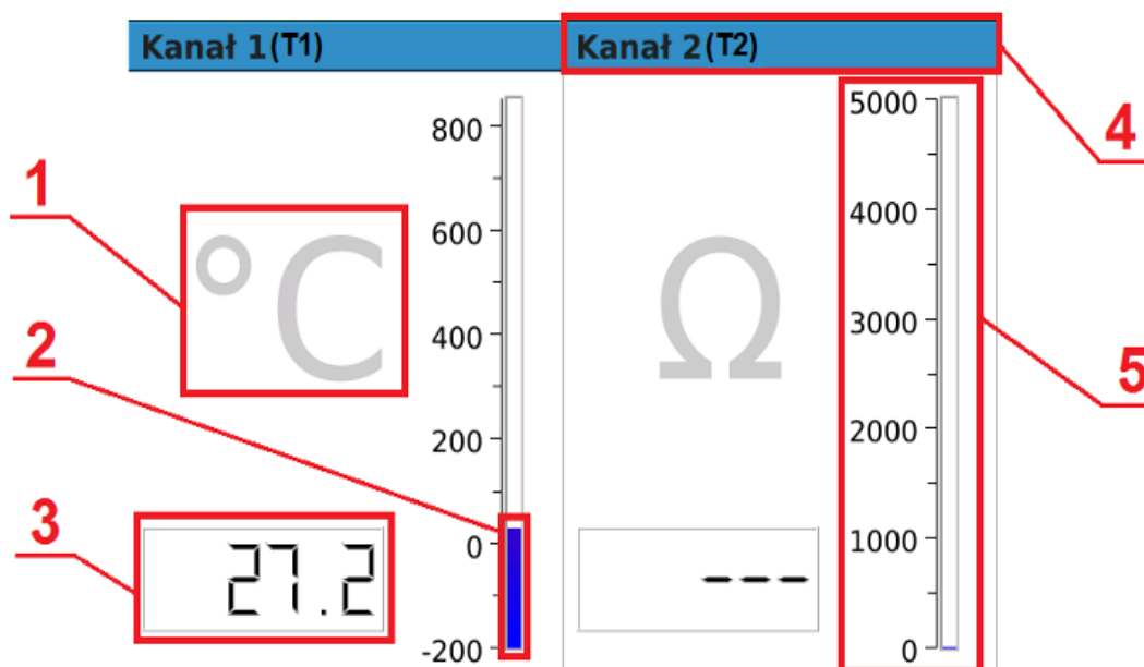
Rys. 75. Temperatura/rezystancja.
