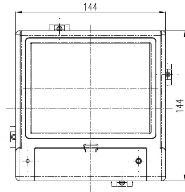
Rys. 21. Wymiary - przód.
