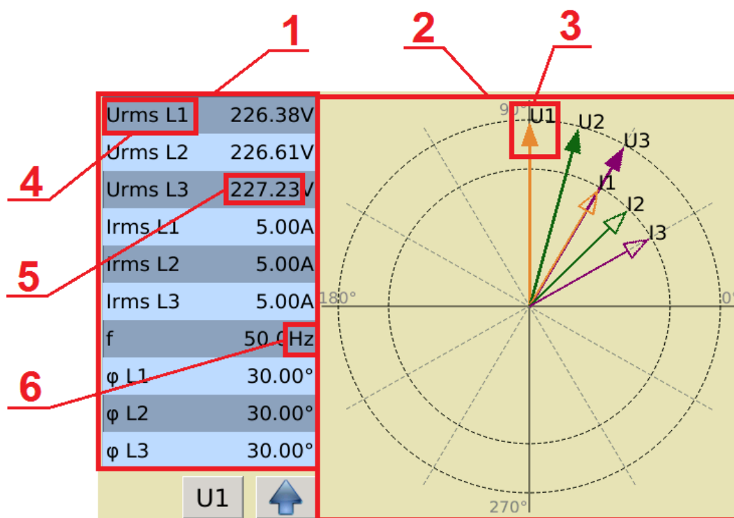
Rys. 73. Diagramy wektorowe.
