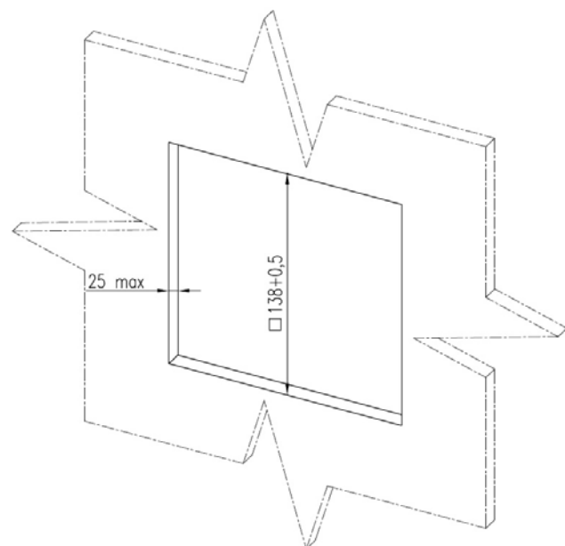
Rys. 23. Wymiary – otwór montażowy.
