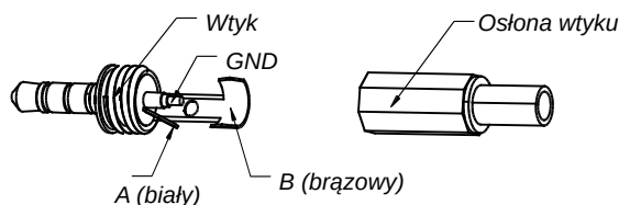
Rys. 19. Połączenie odbiornika STR.
