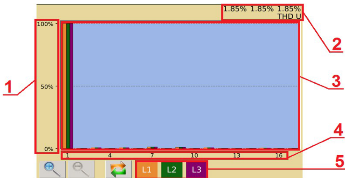
Rys. 68. Harmoniczne.
