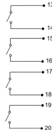
Rys. 13. Wyjścia przekaźnikowe.
