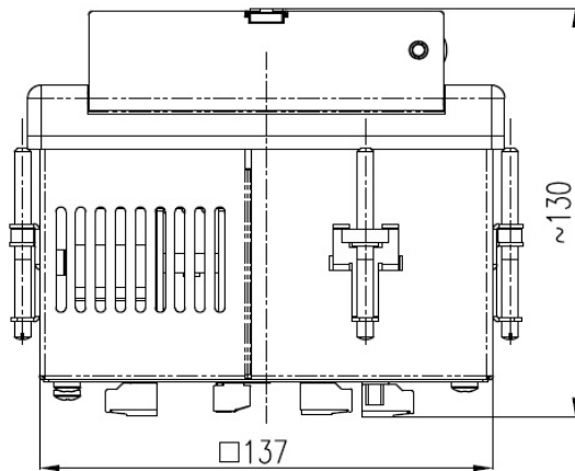
Rys. 20. Wymiary - dół.
