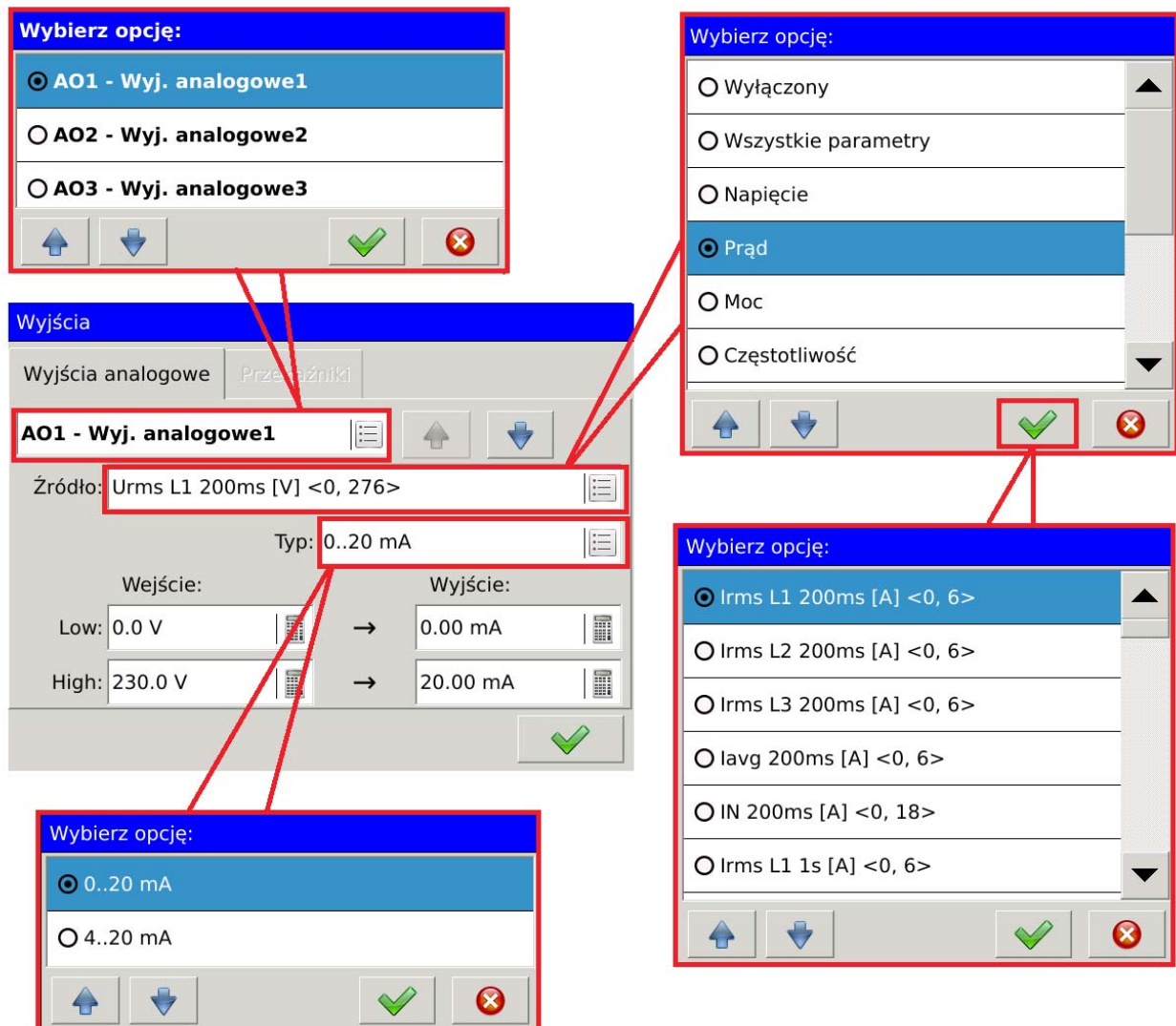
Rys. 150. Wyjścia - wyjścia analogowe.
